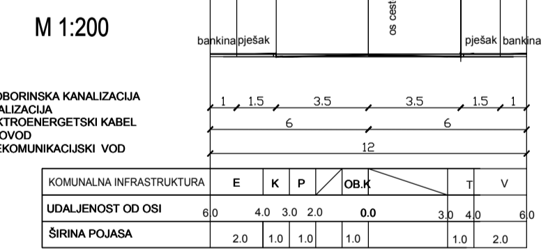
KARAKTERISTIČAN POPREČNI PRESJEK A M 1:200
