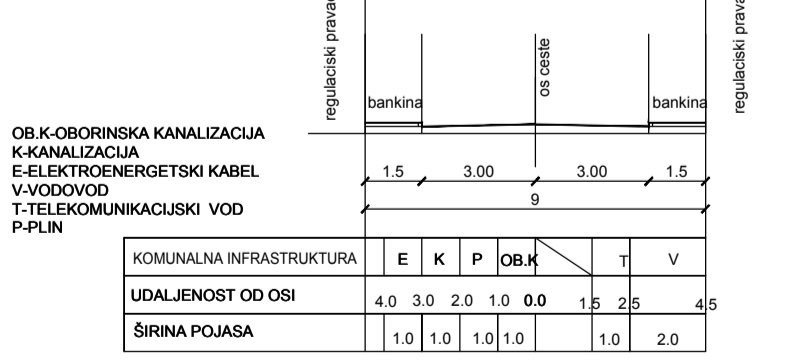
KARAKTERISTIČAN POPREČNI PRESJEK B M 1:200
