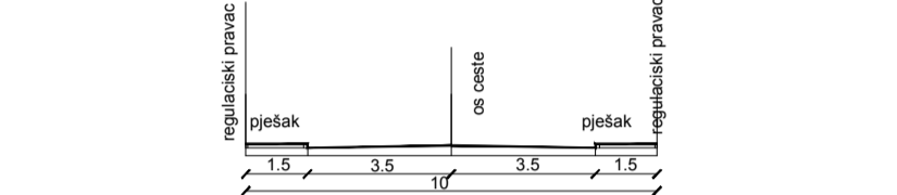
KARAKTERISTIČNI POPREČNI PRESJEK B-B
